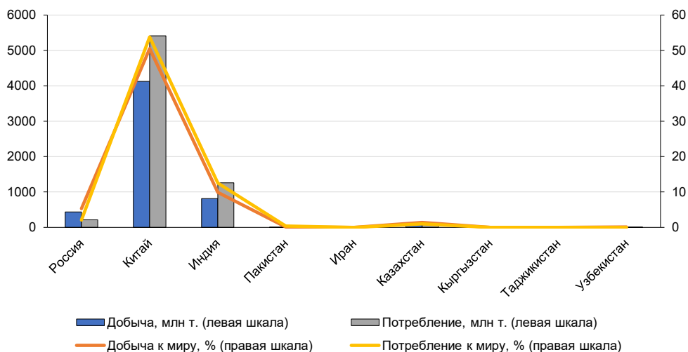
Рисунок 11. Добыча и потребление угля в странах ШОС
