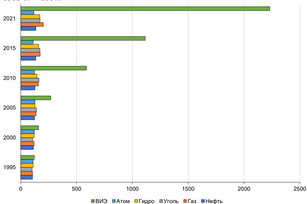
Рисунок 2. Темпы роста потребления энергии по видам источников, 1991 г. = 100%
