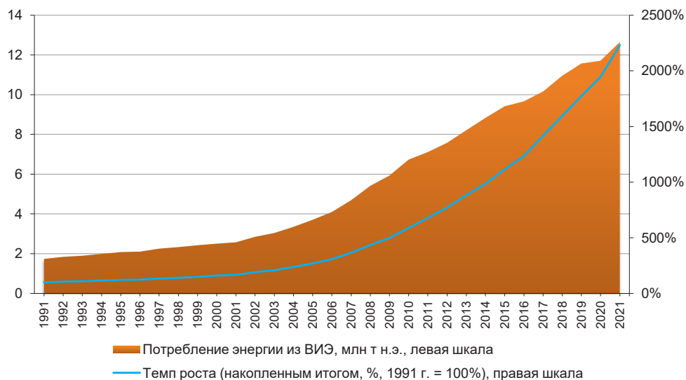
Рисунок 3. Динамика потребления энергии из ВИЭ и темпы роста
