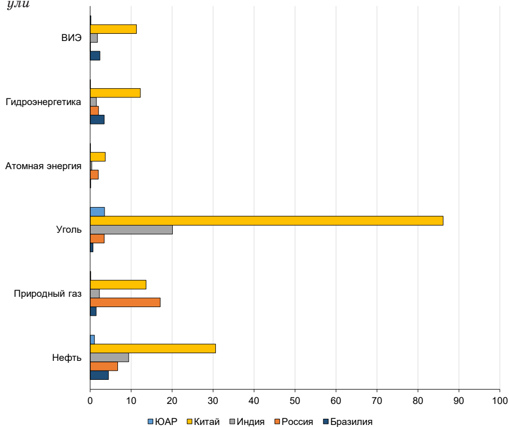
Рисунок 12. Энергетический баланс государств БРИКС в 2021 г., эксаджоули
