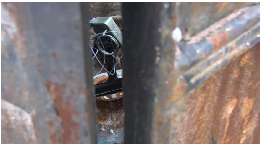
Фугас, установленный на неизвлекаемость с помощью запала от ручной гранаты.
